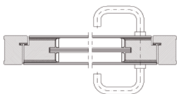
Horizontalschnitt PLANDOOR
